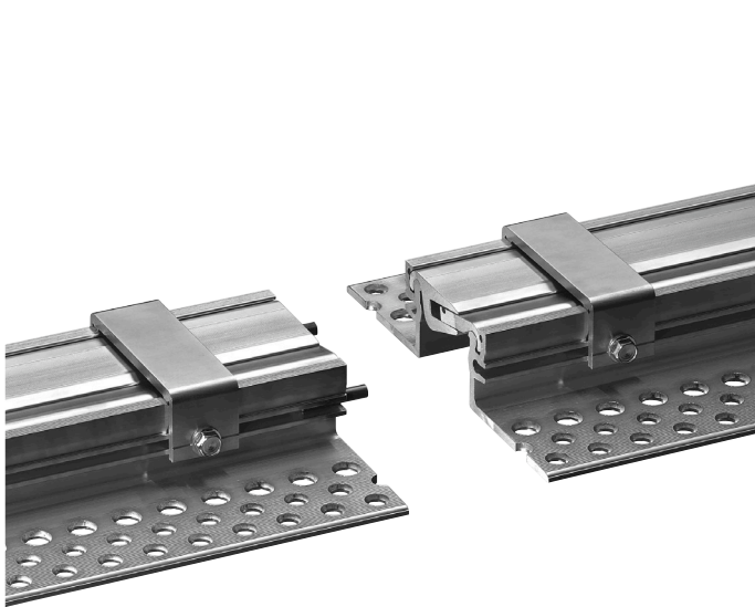
FS 75/42 (einteilige Profilkonstruktion)
